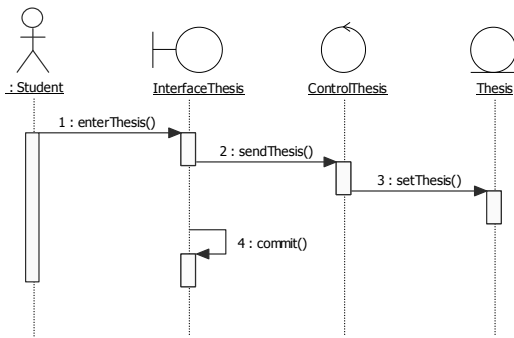
รูปที่ 3 แผนภาพซีคอนซ์ส่วนการอัปโหลดไฟล์เข้าสู่ระบบ
